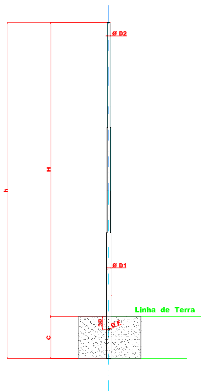
CPR E Poste Reto Engastado CALEDONYA
