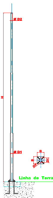
CPR E Poste Reto Flangeado CALEDONYA
